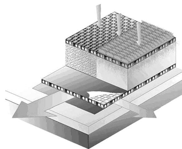
Pavimento vegetado o gravilla estabilizada
