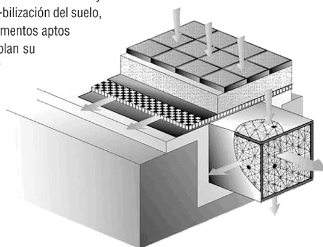
Adoquines con juntas permeables
